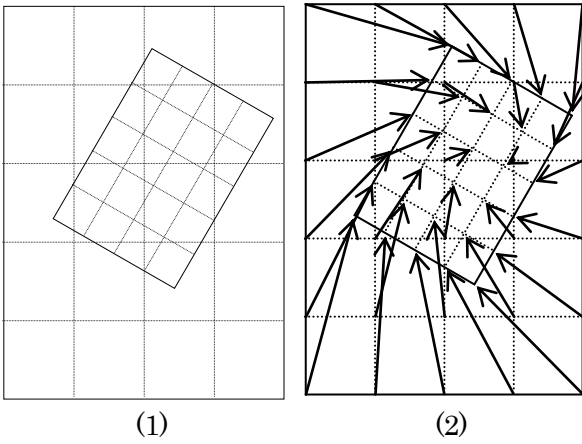
図4. 対応する格子間に矢印を入れる.
