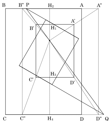
図 11. 上下の辺がそろおう.
