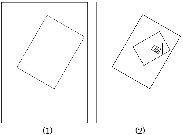
図3. 相似変換の不動点
