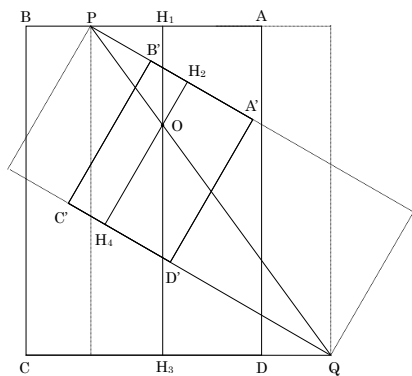
図10. 直線 PQ 上に回転中心をとる．
