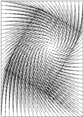
図5. パソコンで描いた相似変換
