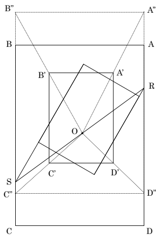
図 13. 左右の辺がそろふ.
