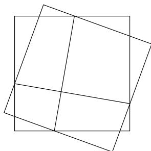
図1. 合同変換の不動点
