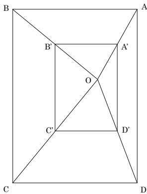
図6. 相似の中心
