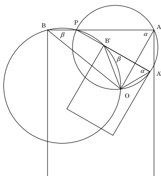
図7. 相似図形を用いる (解1)
