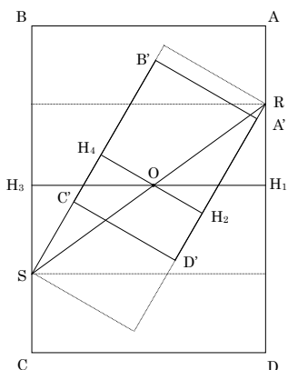
図 12. 直線 RS 上に回転中心をとる.
