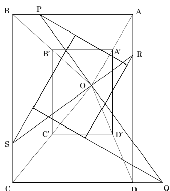
図 14. 上下，左右の辺がそろう．
