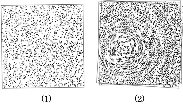
図2. ランダムドット・パターン
