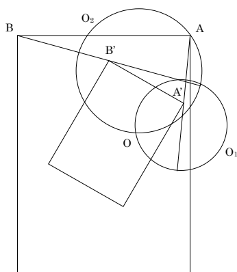
図8. アポロニウスの円を用いる (解2)
