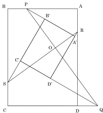
図9. コンパスを使わない方法 (解3)
